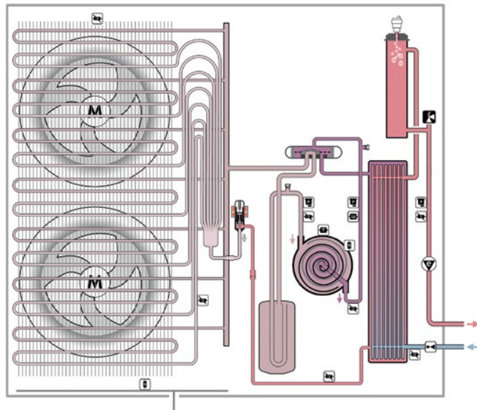
Prikaz komponenata kod modela VWL 125/6 i VWL 155/6
