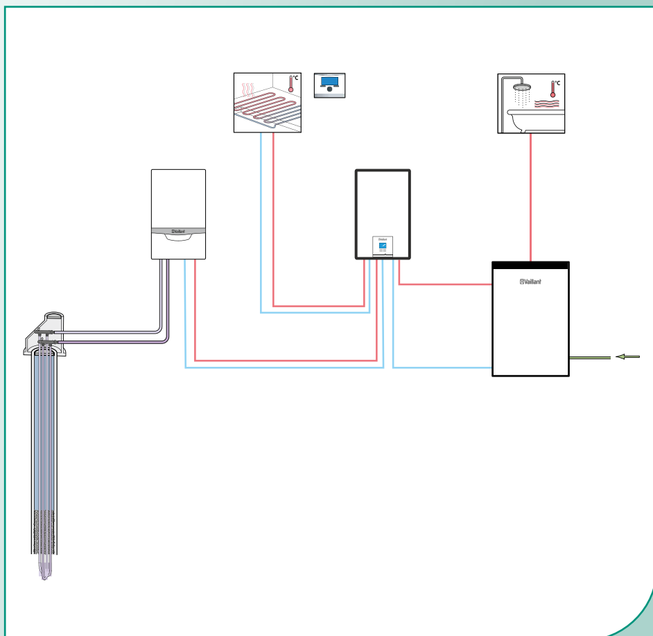
Hibridni sustav - dizalica topline zadužena je za grijanje i hlađenje dok se kondenzacijski uređaj koristi za potporu grijanju i pripremu PTV
