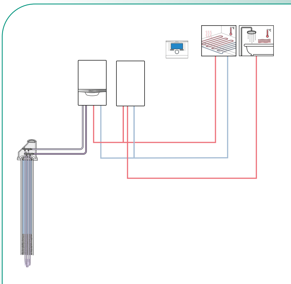
Monoenergetski sustav - dizalica topline zadužena je za grijanje, hlađenje i pripremu PTV u kombinaciji sa zidnim električnim modulom
